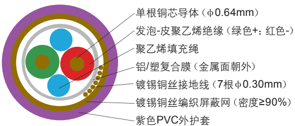
型号: TKPC 规格: 1 \times 2 \times 22\text{AWG}
