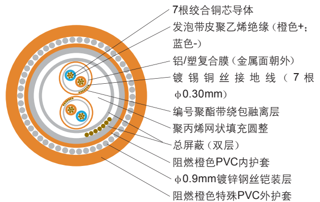
型号: TKFFAR-A 规格: 2 \times 2 \times 0.8\text{mm}^2 (18AWG)
