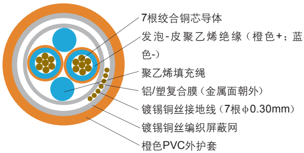
型号: TKFF-A 规格: 1 \times 2 \times 0.8\text{mm}^2 (18AWG)
